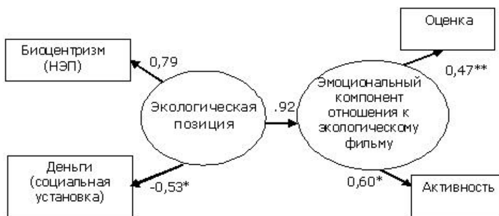
Рисунок 2. Модель влияния экологической позиции на эмоциональное отношение к экологическому фильму ( \chi^2/df=0,59/1 ; p=0,44 ; RMSEA 0; GFI 0,995; AGFI 0,95; связи значимы при p<0,001 , кроме * p<0,01 и ** p<0,05 )
